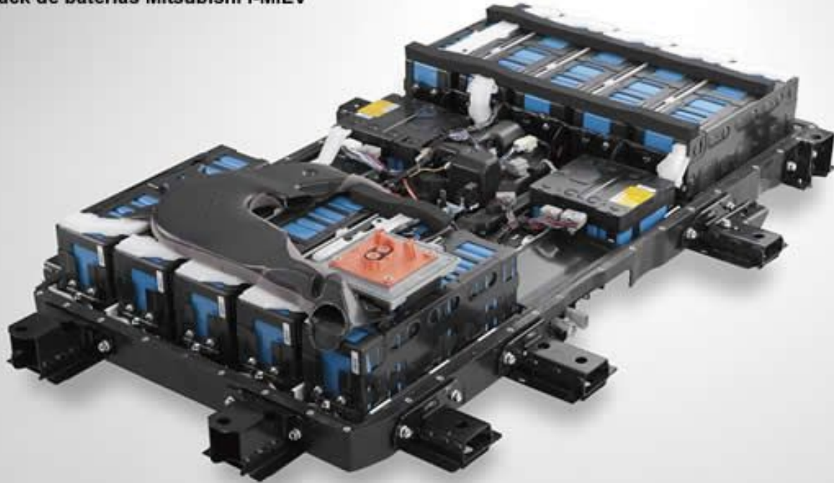
Pack de baterías Mitsubishi i-MiEV
