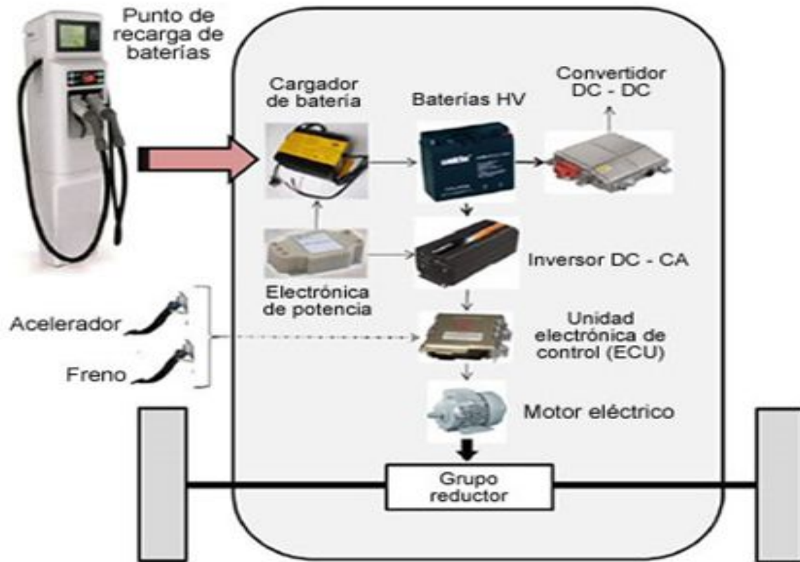
Esquema de componentes de un coche eléctrico.
