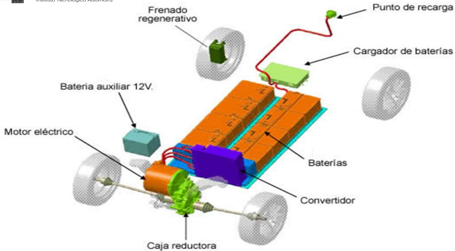
Esquema básico de un coche eléctrico
